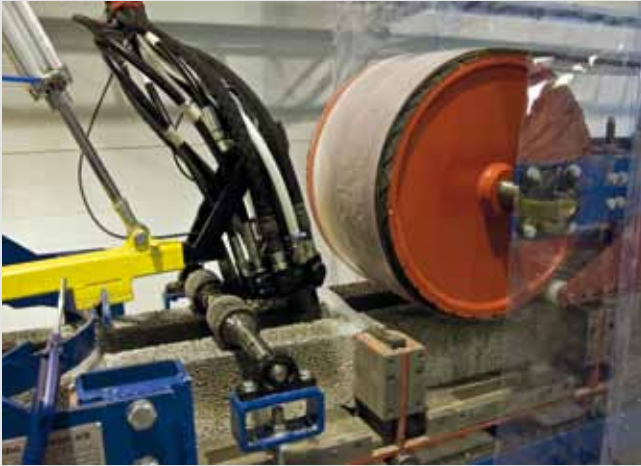
Aufschäumungsposition für das Einspritzen von PU-schaum
